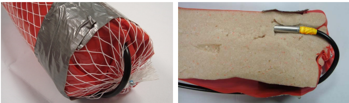
Abb. 1 und 2: Stirnseitige Anbringung der Sprengkapsel Nr. 8 RICHTIG!
